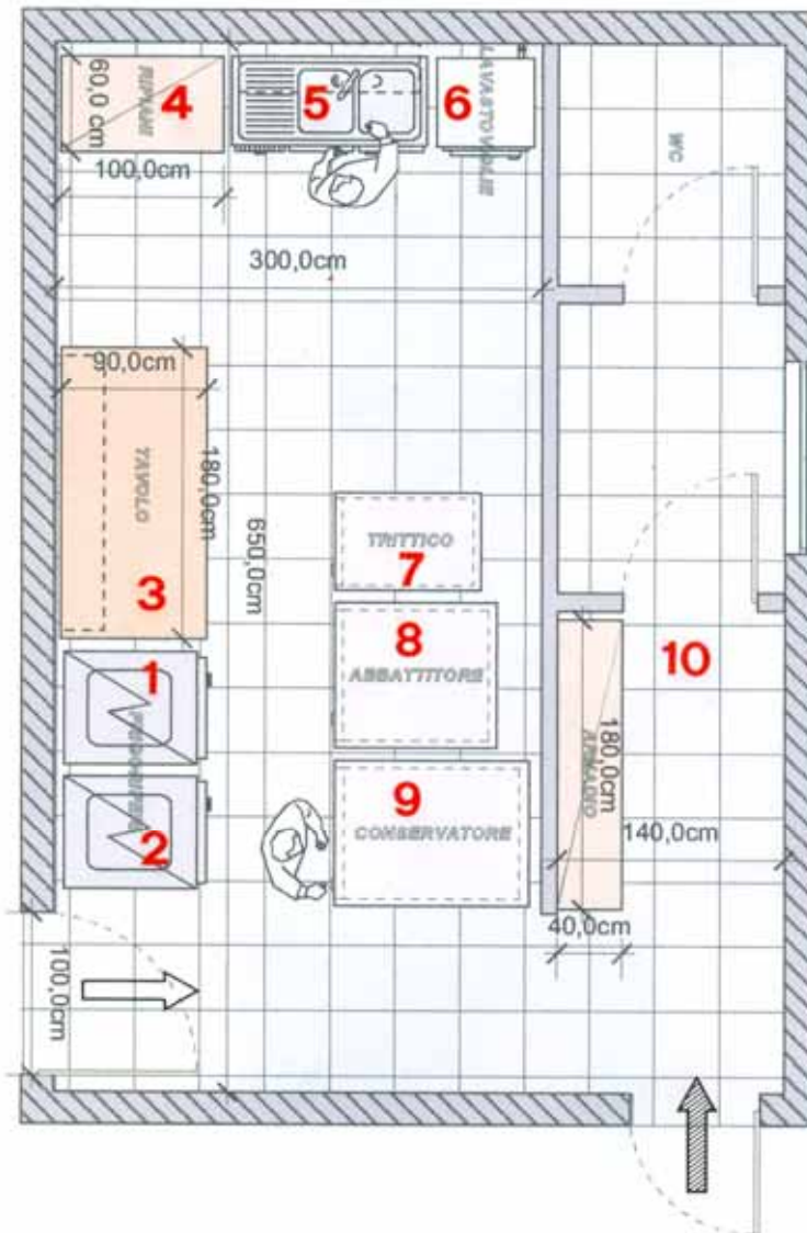
Layout Laboratorio di 30 mq scala 1:50
